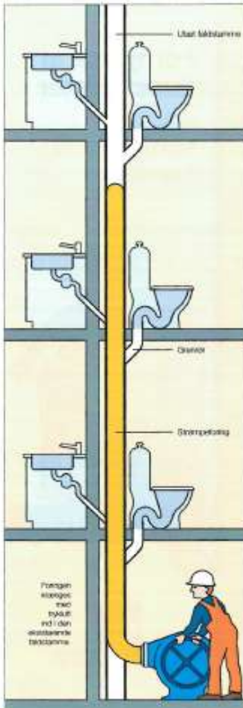
Figur 6.9. Installation af en strømpeføring. Posen indføres med trykluft, og hærdes ved at tilføre varme/lys mens posen holdes under tryk
